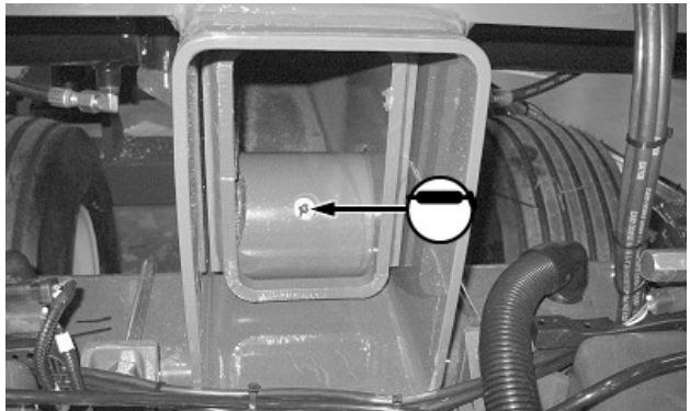
Валок задньої центральної зчіпки
