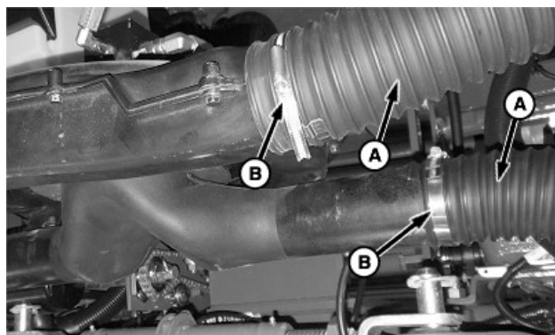
A—Гнучкі шланги B—Шлангові хомути
