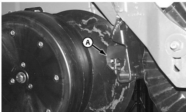
A—Скребок для важких умов експлуатації
