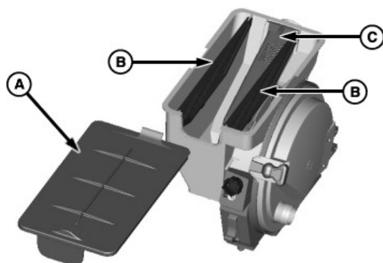
A—Кришка B—Дільники з ситами C—Розвантажувальна трубка
