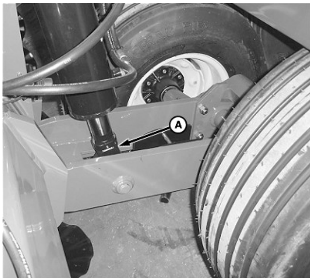
A—Вилка
