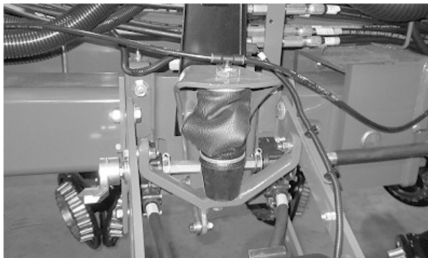
Нерозтягнута пневмопругина
