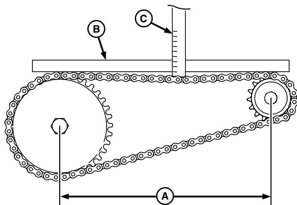
Приводний ланцюг без натяжного шківa
