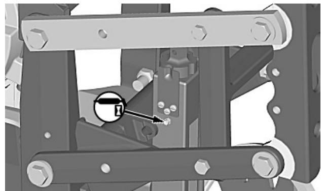
Регулювальна штанга очищувача рядків, змонтованого на апараті
