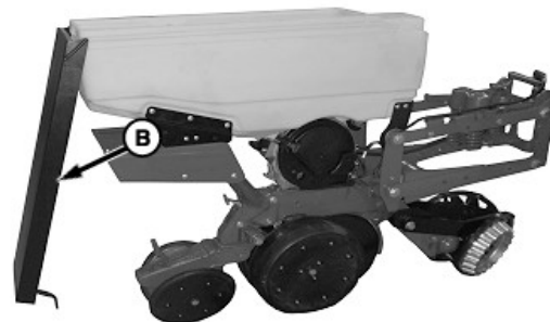
Насіннєвий бункер місткістю 106 л (3 буш.)
