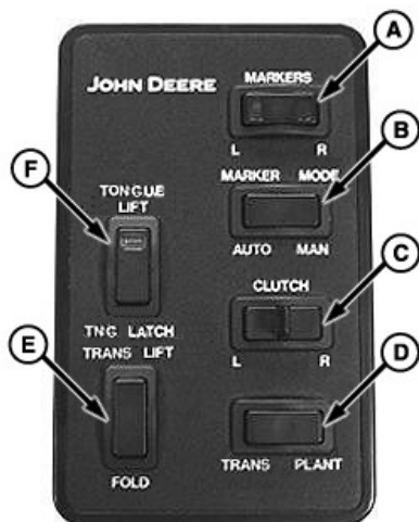
A—Перемикач маркерів B—Перемикач режиму маркера C—Перемикач зчеплення D—Перемикач посіву/транспортування E—Перемикач підйому/складання для транспортування F—Перемикач підйому дишла/засувки дишла
