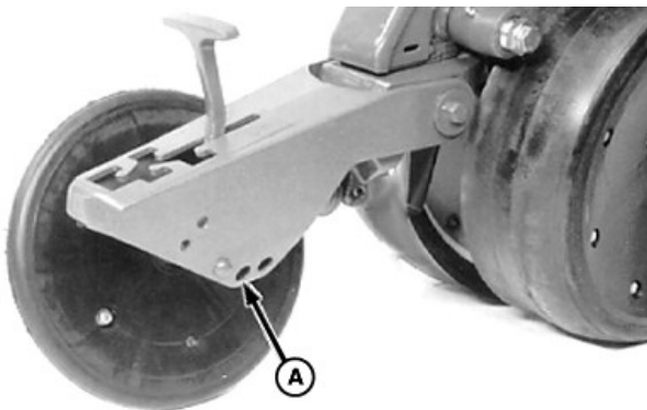
A—Задній отвір
