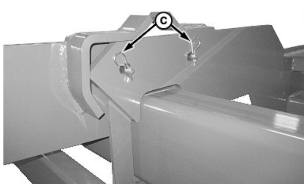
A—Транспортний хомут B—Штифт (2 шт.) C—Пружинний шплінт (2 шт.)
