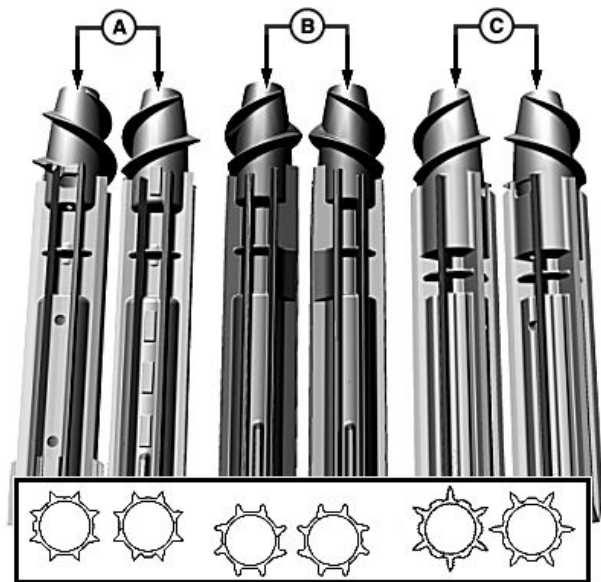
A—Rolos Espigadores da Faca Oposta B—Rolos Espigadores de Ranhuras Retas C—Rolos Espigadores da Faca de Entrelaçamento
