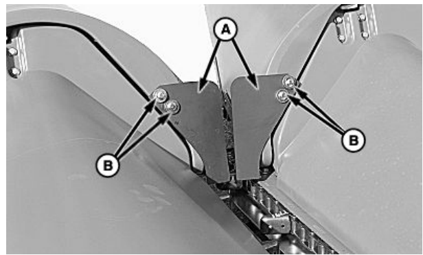
A—Protetores de Espigas
