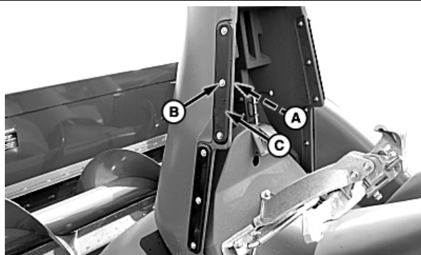
A—Nakrętka i podkładka B—Śruba i podkładka
