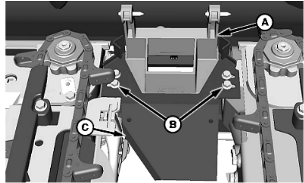
A—Podpora osłony podbieracza B—Śruby (4 szt.)
