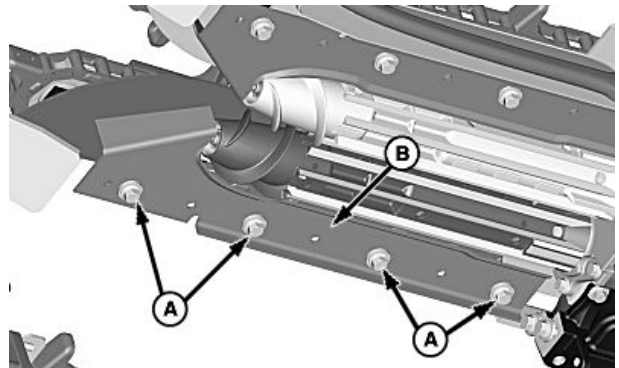
B—Couteau déboureur (2)
