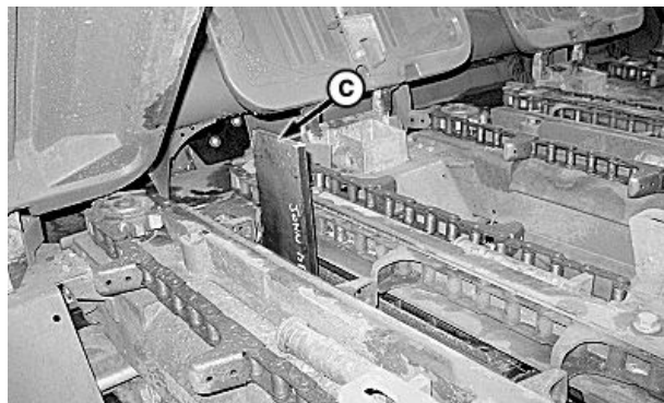
Dépose de l'écrou de fixation gauche
