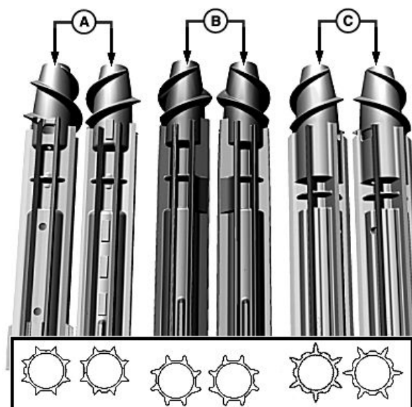
A—Rouleaux preneurs à lames symétriques B—Rouleaux preneurs cannelés droits
