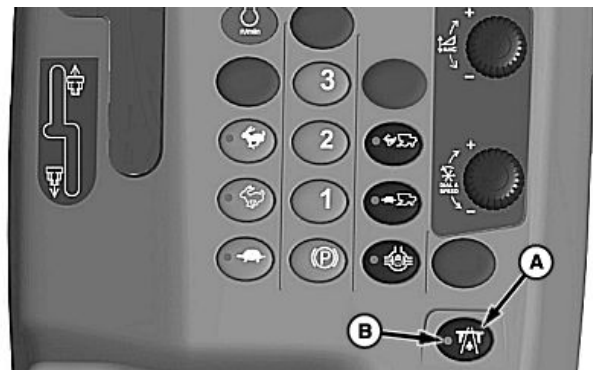
Vista de una cosechadora de la Serie S
