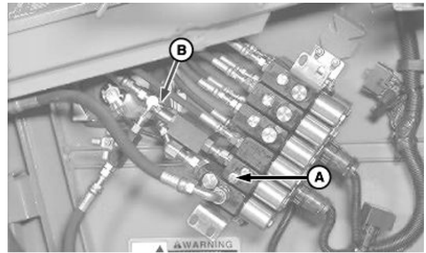
Комбајни од серија 50 STS
