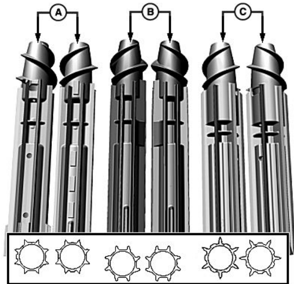
A—Rolos Espigadores da Faca Oposta B—Rolos Espigadores de Ranhuras Retas
