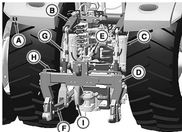
Součásti zadního závěsu
