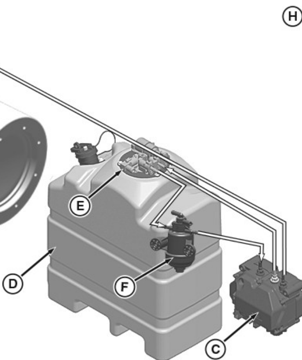
Systém SCR
