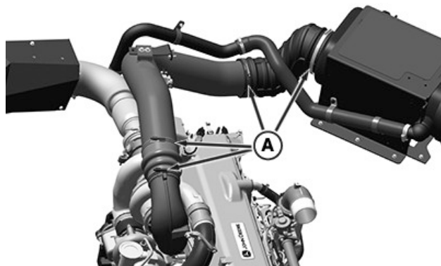
Motor s dvoufázovým turbodmychadlem
