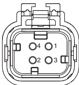
Označení pinů analogového video konektoru
