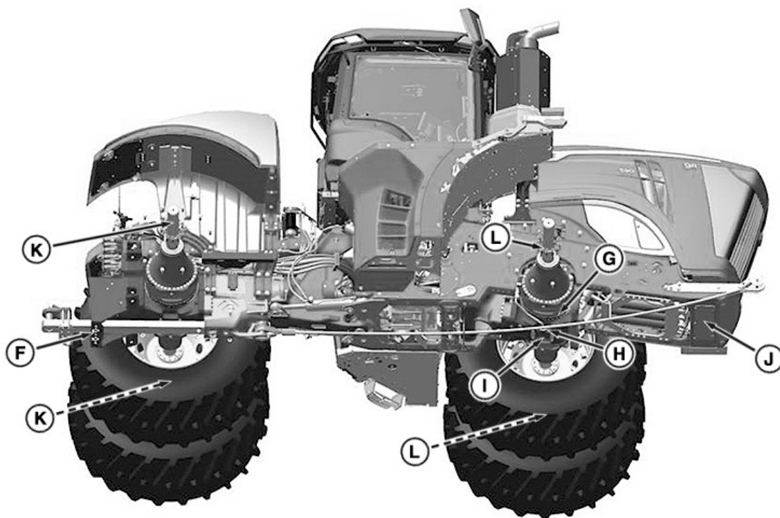
Zvedací body (spodní strana se spodním závěsem [zemědělství])
