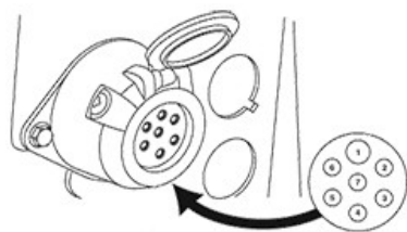
Schéma zásuvky
