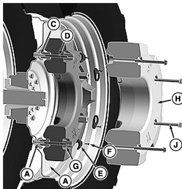
Přídatné závaží kol – obrázek 2
