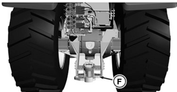
Podpěrné body (zadní spodní závěs)
