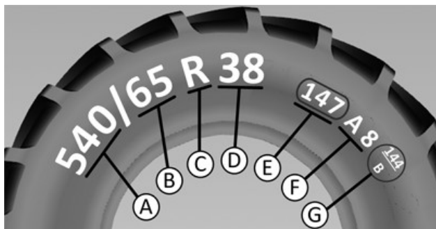
Příklad informací výrobce na boční stěně pneumatiky
