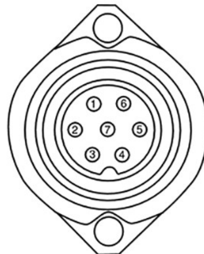
Schéma zásuvky ISO 11786
