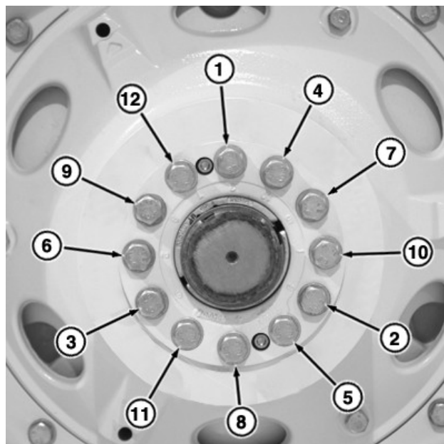
RXA0090157—UN—08AUG06 Pořadí utahování: Sestava náboje hnacího kola se zvýšenou odolností s dvojitým zkosením
