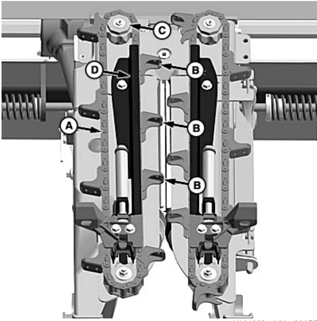
A—Cadena recogedora B—Aletas de la cadena con el menor espaciado (se usan 3) C—Rueda dentada motriz D—Guía de cadena
