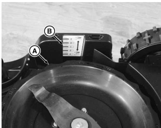
A—Protección de la hoja niveladora B—Etiqueta de altura de corte
