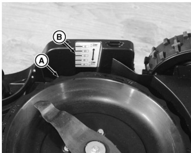
A—Messerschutz
