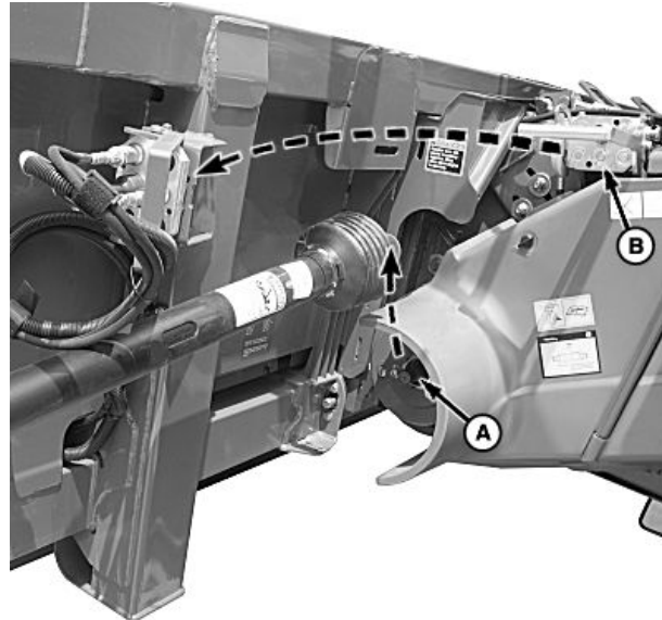
A—Wał przenośnika pochylego B—Wielozłätze
