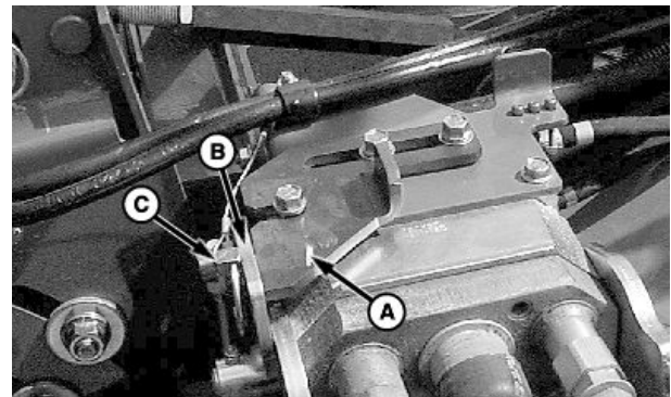
Maszyny wyposażone w przesuwaną płytę blokującą
