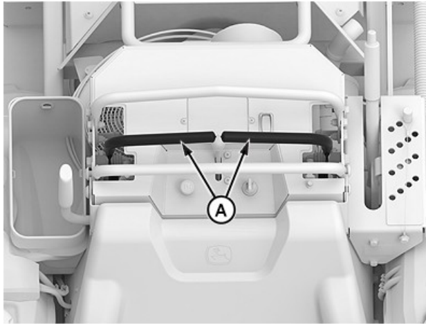
APY580204—UN—28JUL23 Leviers de commande de déplacement (A) illustrés en position point mort.
