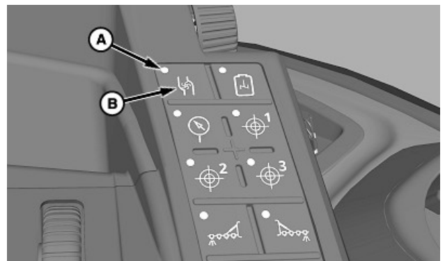
A—Luz testigo B—Interruptor de activación del sistema hidráulico
