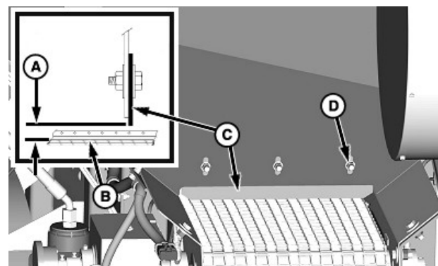
A—Apertura del portón de alimentación B—Suelo del transportador C—Portón de alimentación D—Tuerca (se usan tres)
