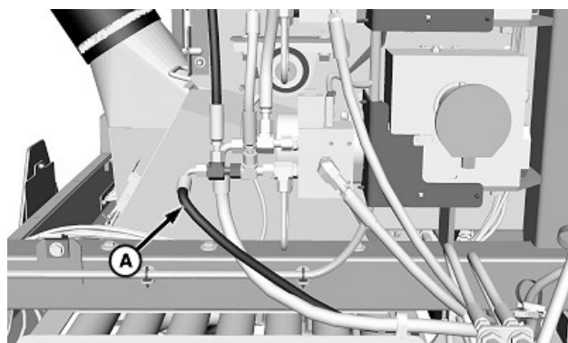
A—Manguera hidráulica de 1260 mm (49.6 in)
