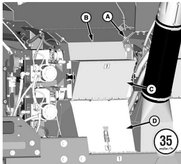
A—Tornillo (se usan dos) B—Cubierta del transportador C—Embudo superior del transportador D—Embudo inferior del transportador
