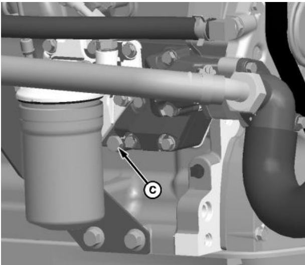
A—Tapón de llenado B—Vaciado del radiador C—Tapón del bloque
