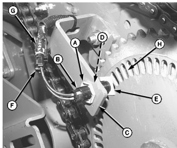
Captador magnético de velocidad del molinete
