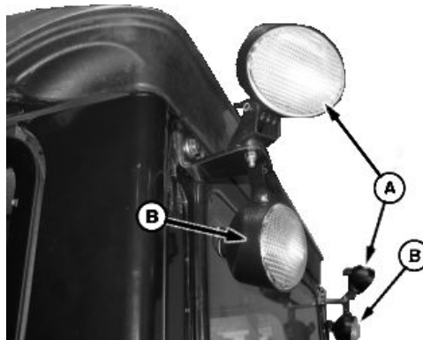
A—Faros de trabajo superiores B—Faros de trabajo inferiores
