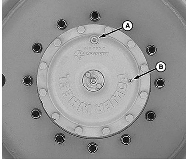
A—Tapón de llenado/vaciado
