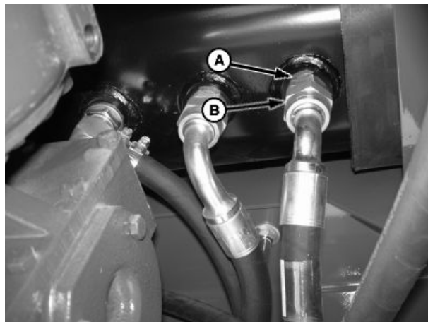
A—Racor
