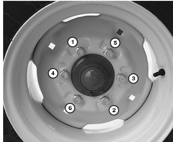
Tornillos de rueda trasera
