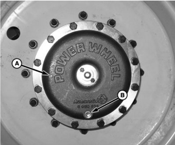
A—Tapón de inspección B—Tapa de llenado/vaciado
