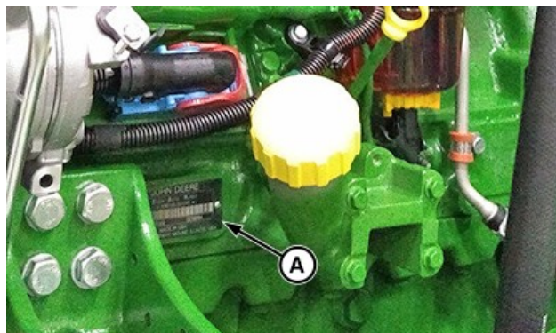
Placa del número de serie del motor (A) (piezas retiradas para mayor claridad)
