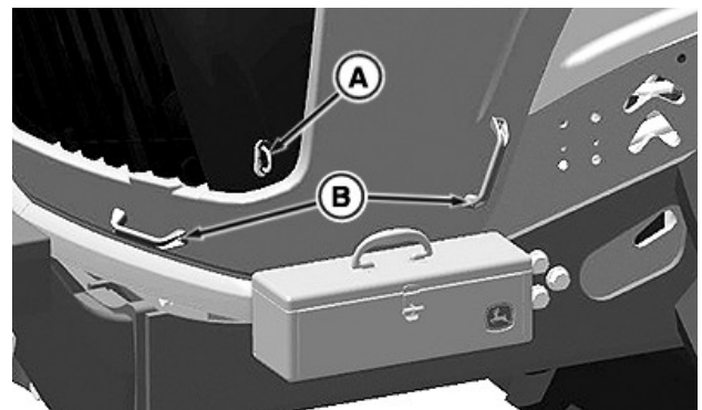
Eliberarea capotei și mânerul capotei
