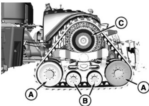
Șenilă lată
