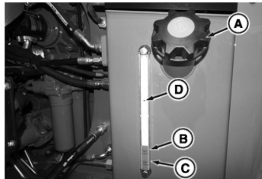
Indicator de nivel al rezervorului hidraulic
