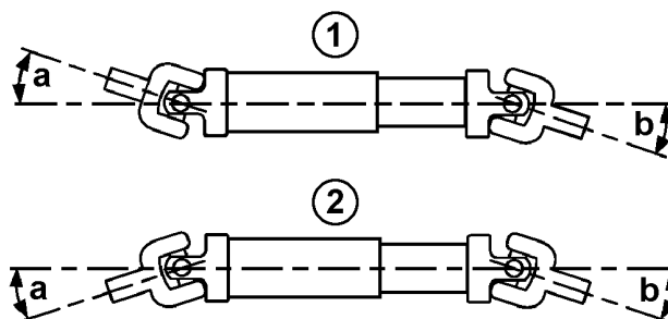
Articulația de la arborele de antrenare
