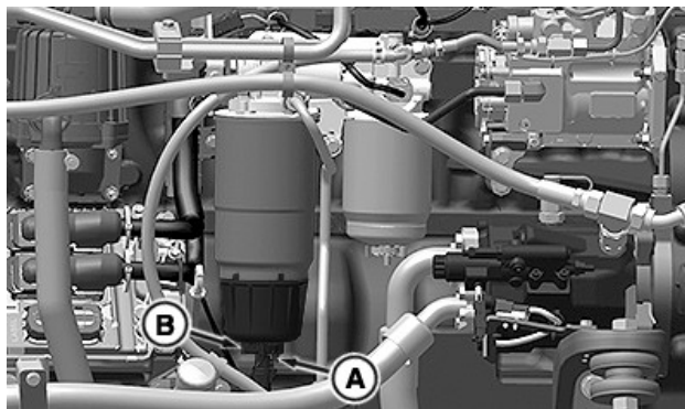
RXA0180389—UN—06NOV20 Filtru de carburant motor de 13,6 l
