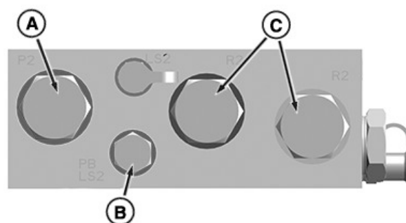
Porturile blocului de putere hidraulică externă—mijloc/sus (dacă există)
