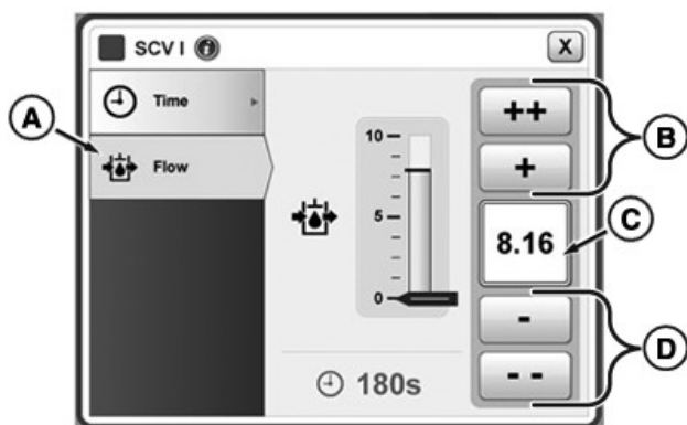
RXA0131683—UN—28MAR13 Debitul de detentă SCV
