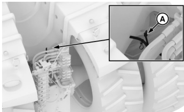
Conectarea cablajului senzorului de tracțiune
