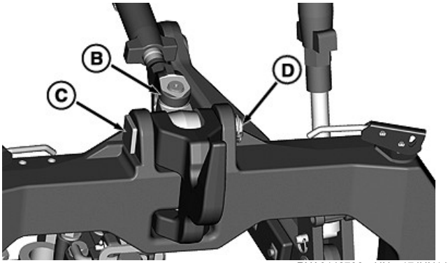
Bară centrală
