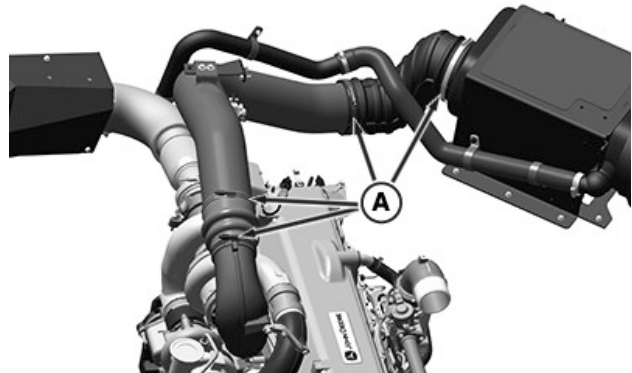
Motor cu turbosuflantă cu două trepte
