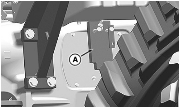
RXA0188671—UN—23FEB23 Blokada układu kierowniczego w miejscu przechowywania (lewa strona)
