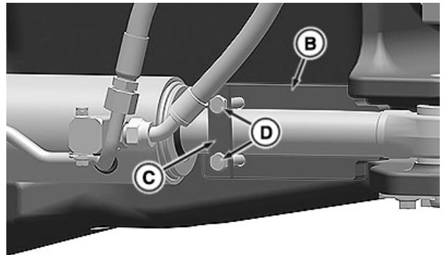
RXA0188672—UN—23FEB23 Zamontowana blokada układu kierowniczego (lewa strona)
