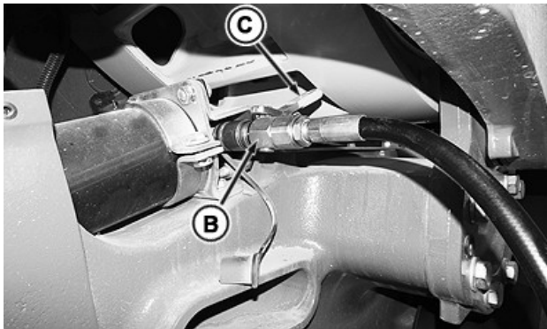
Przewód napinania/luzowania gąsienic
