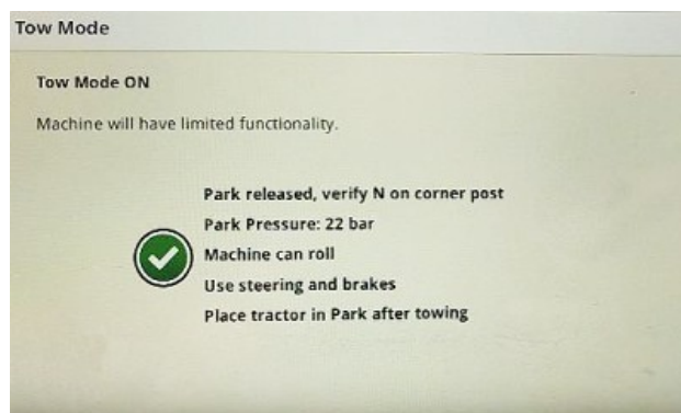
Ciśnienie postojowe trybu holowania
