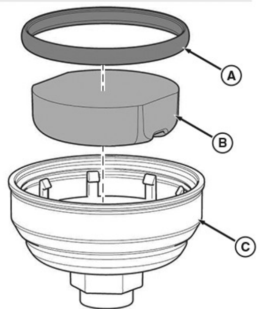
RG30726—UN—08AUG18 Componenti dell'alloggiamento del filtro
