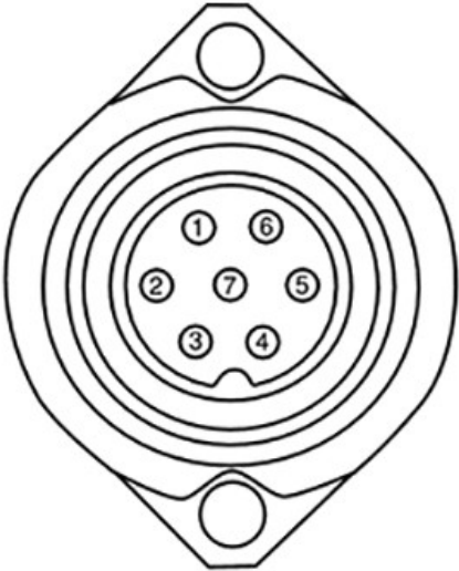
Schema della presa ISO 11786
