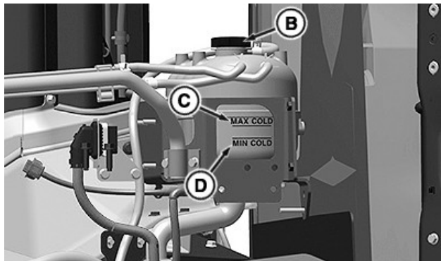
RXA0180388—UN—06NOV20 Двигатель объемом 13,6 л
