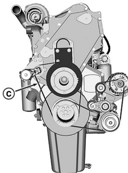
Схема расположения приводного ремня вентилятора на машине с двигателем объемом 13,6 л
