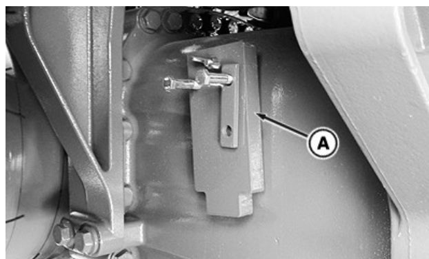
Блокирующий ограничитель гидроцилиндров рамы с левой стороны в положении хранения
