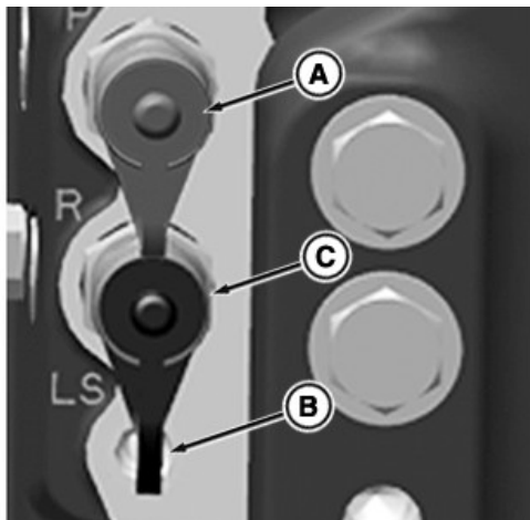
Муфта Power-Beyond — литые компоненты навески
