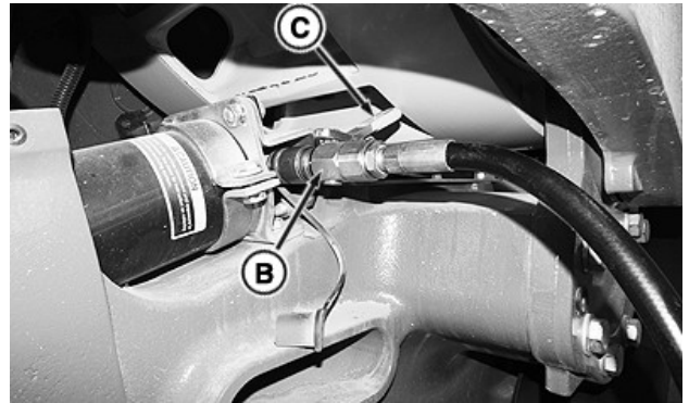
RXA015271—UN—20OCT15 Шланг для увеличения/ослабления натяжения гусеничных лент
