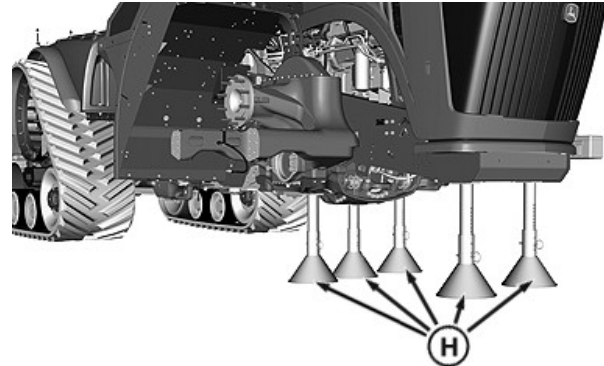
Установка опорных стоек JT07211
