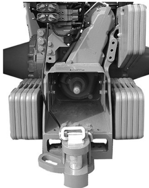
RXA0153814—UN—07SEP16 Maximální konfigurace závaží s vývodovým hřídelem
