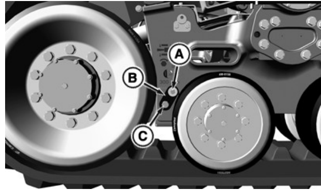
Außenseite des Raupenfahrwerk-Rahmens
