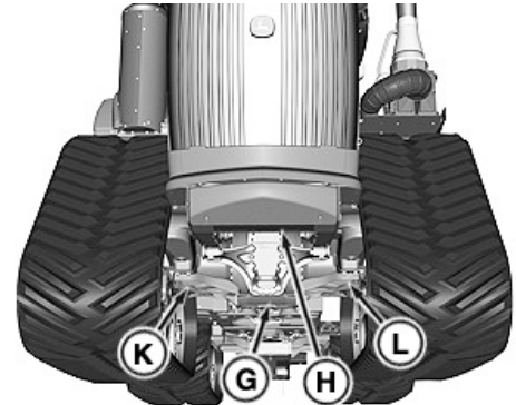
Hebepunkte (vorne)
