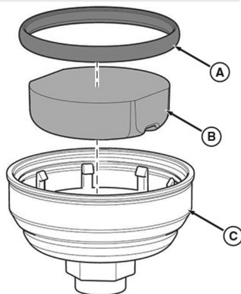
Filtergehäuse – Komponenten
