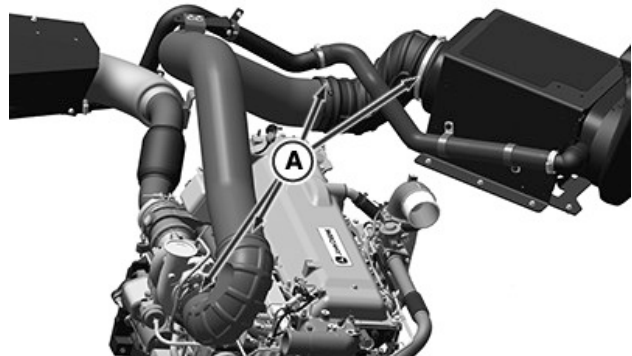
Einstufen-Turboladermotor
