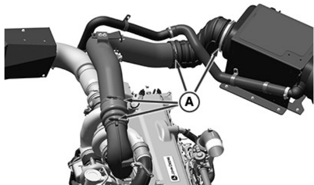
Doppel-Turbolader-Motor
