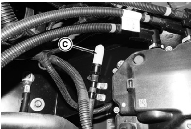
RXA0142031—UN—03JUN14 Der EntlüftungsfILTER (C) des DEF-Tanks befindet sich im Batteriefach über der DEF-Dosiereinheit.
