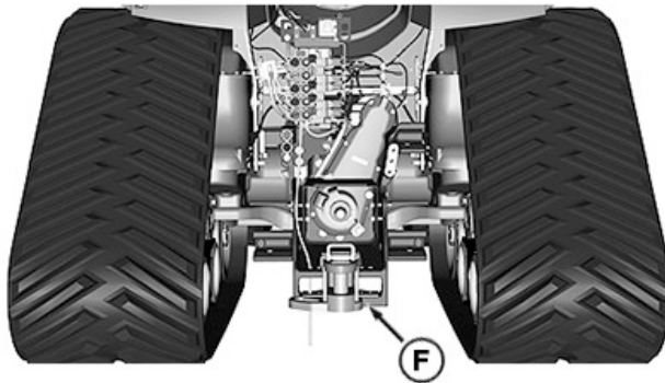
Hebepunkte (hinteres Zugpendel)
