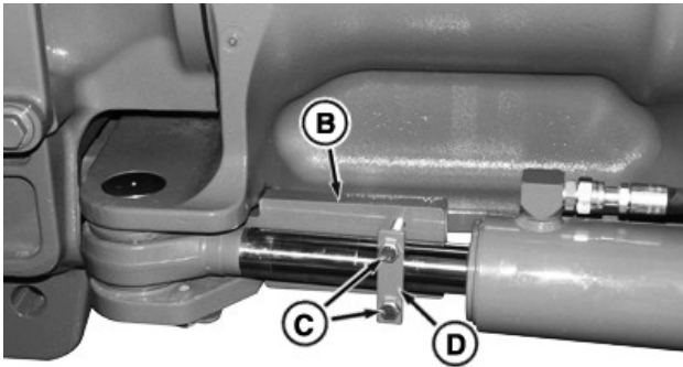
RXA0160311—UN—27JUL17 Verrou d'articulation monté
