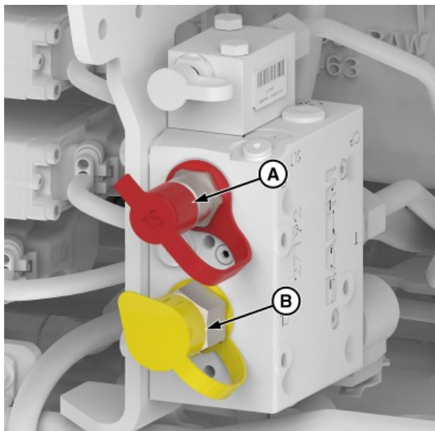
Raccords de frein hydraulique de remorque
