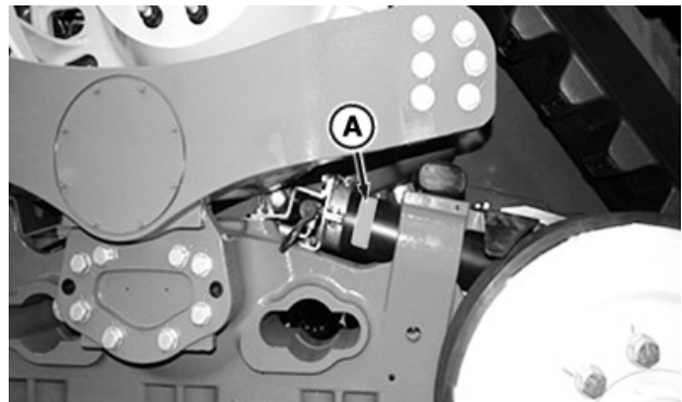
A—Autocollant d'accumulateur (chenilles gauche, droite, avant et arrière)
