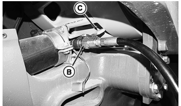
Flexible de tension/détente de chenille
