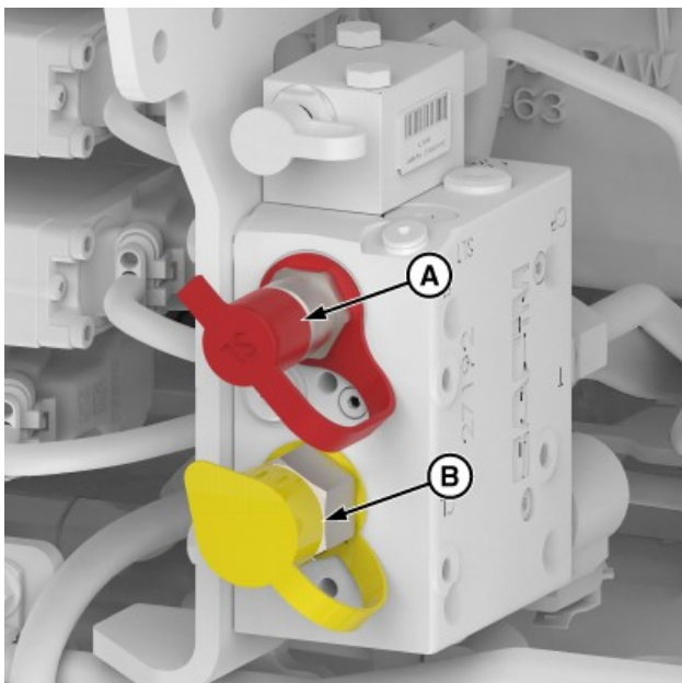
Гидравлик тиркама тормози муфтлари
