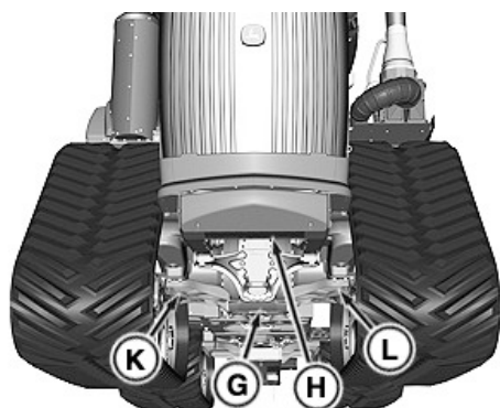
Кўтариш нуқталари (олд)
