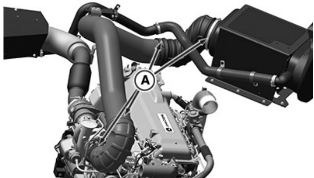
Бир босқичли турбо мотор
