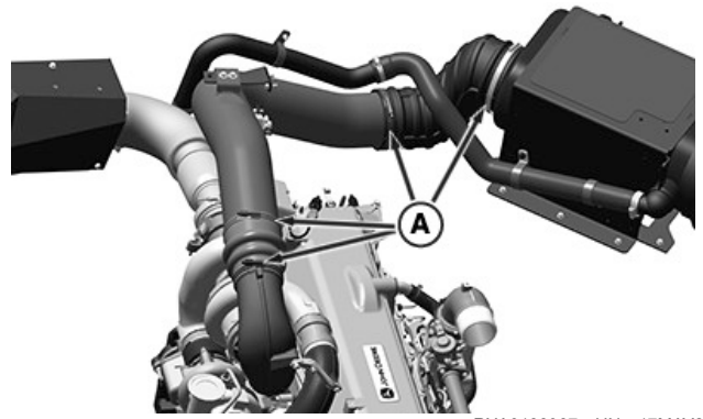
Moteur de turbocompresseur à deux étages
