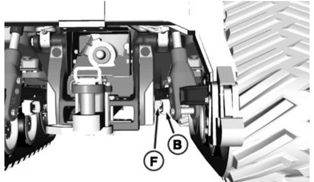
Butée de barre de traction
