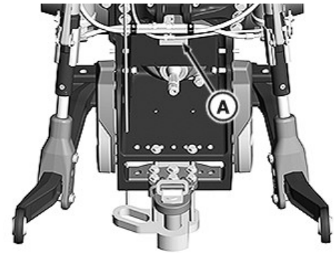
A—Autocollant de prise de force (arrière du tracteur sur le garant de prise de force)
