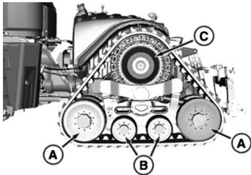
Breite Laufkette RXA0147242—UN—11FEB15
