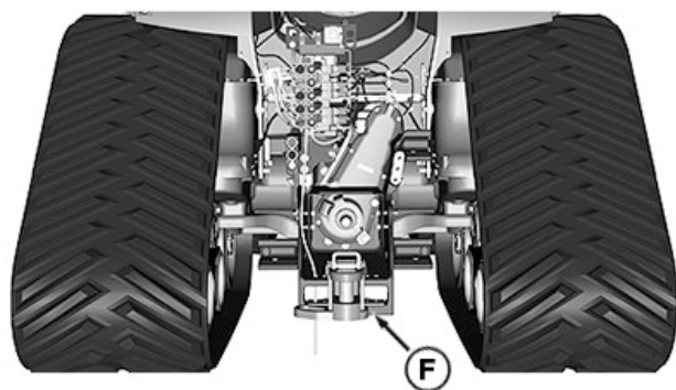
RXA0188405—UN—20DEC22 Hebepunkte (hinteres Zugpendel)
