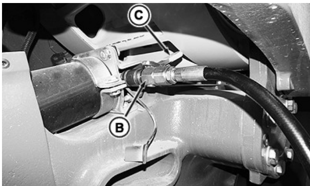
Schlauch zum spannen/entspannen der Kette
