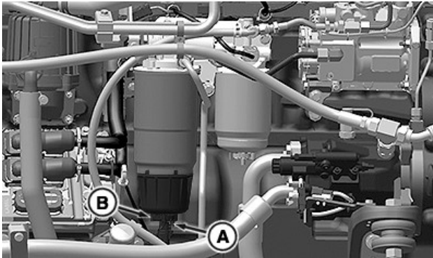
RXA0180389—UN—06NOV20 Kraftstofffilter des 13,6-l-Motors
