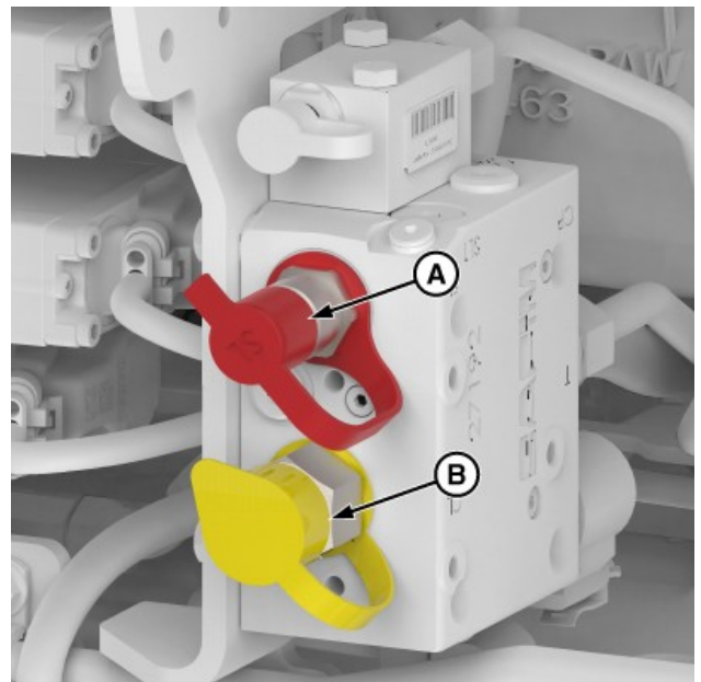
Anschlusskupplung für hydraulische Anhängerbremse
