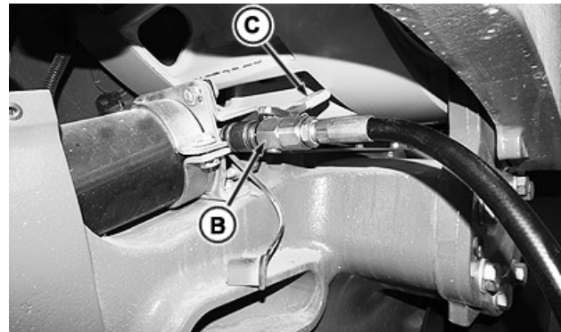
Schlauch zum Spannen/Entspannen der Laufkette
