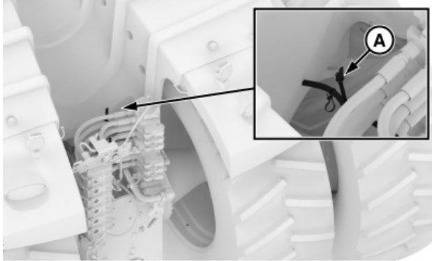
Kabelbaumanschluss des Zugkraftsensors
