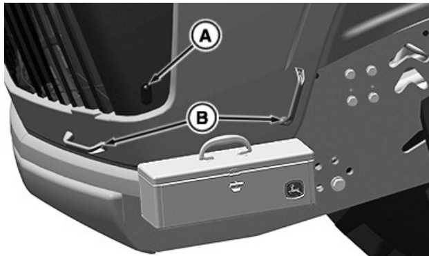
RXA0180141—UN—15OCT20 Entriegelungstaste und Motorhaubengriffe
