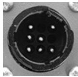
RXA0169821—UN—02AUG19 Stecker nach ISO 11783
