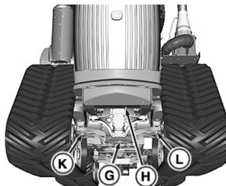
RXA0188406—UN—20DEC22 Hebepunkte (vorne)
