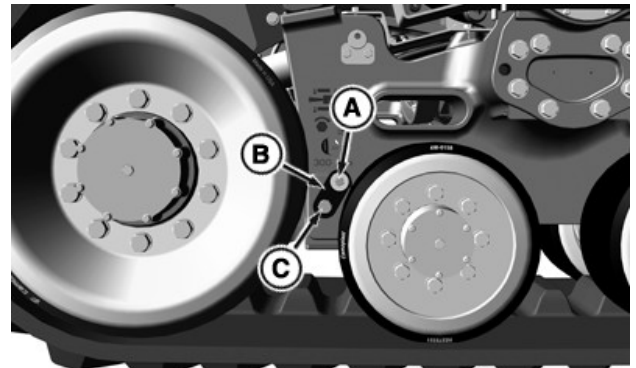
Außenseite des Raupenfahrwerk-Rahmens
