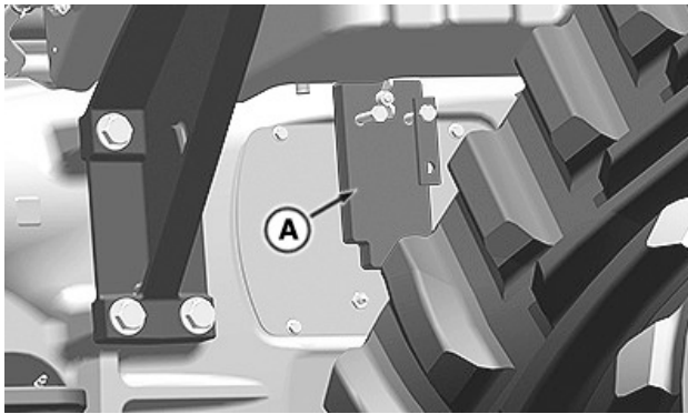
Lenkverriegelung gespeichert (linke Seite)
