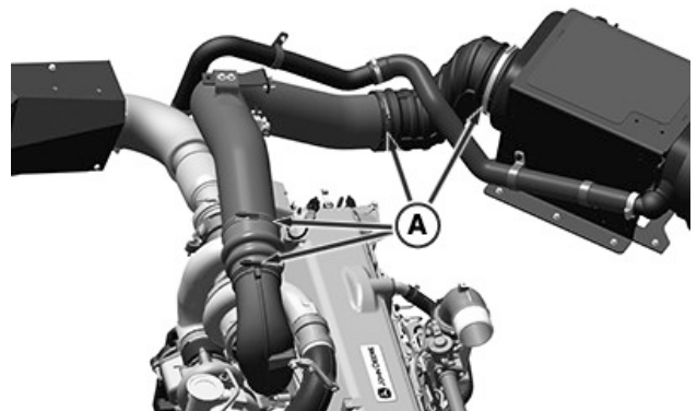
Doppel-Turbolader-Motor
