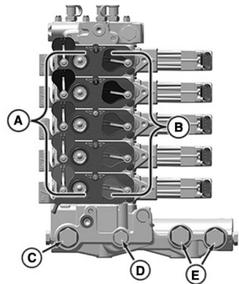
Standard-Durchfluss—Power Beyond in oberer Position
