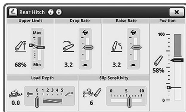
Exemple de relevage arrière
