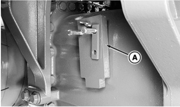
Verrou d'articulation rangé sur le côté gauche
