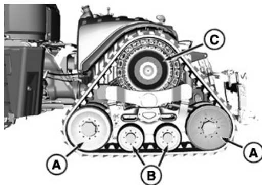
Orugas anchas
