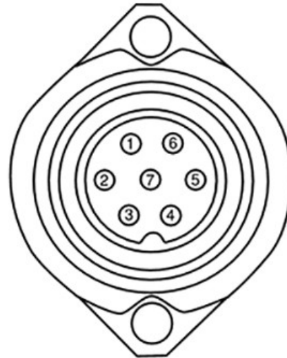
Diagrama de salida ISO 11786
