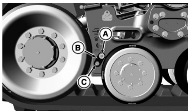
Bastidor de la cadena de oruga exterior
