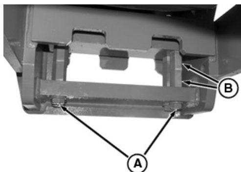
RXA0082010—UN—05JUL05 Instalación del soporte de la barra de tiro más grande de la traílla
