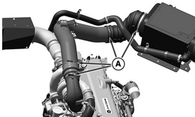
Motor turbo de dos etapas
