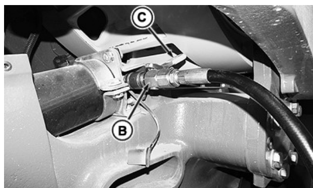
Шланг регулювання натягу/послаблення гусениць
