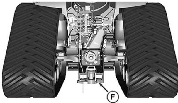
Точки піднімання (задній тягово-зчіпний пристрій)
