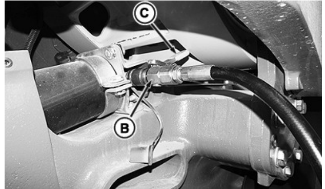
Шланг регулювання натягу/послаблення гусениць
