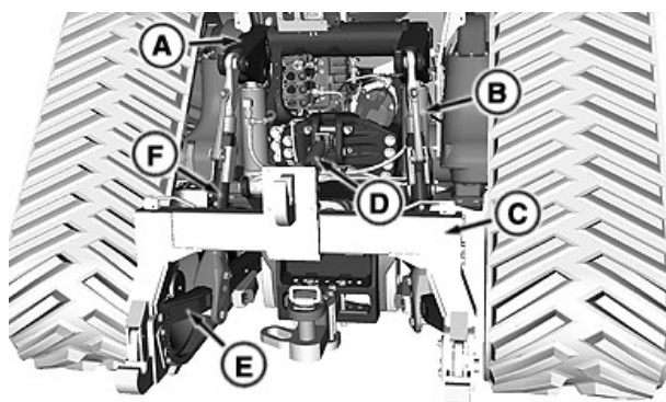
Súčasti závesu
