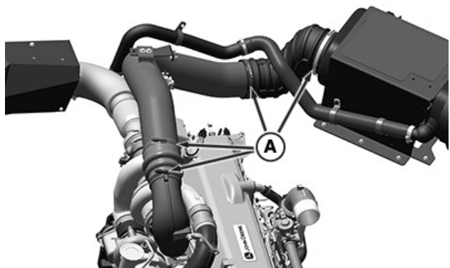
Dvojstupňový turbo motor
