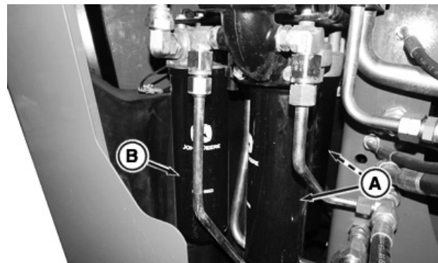
Filtere hydraulickej sústavy a nápravy
