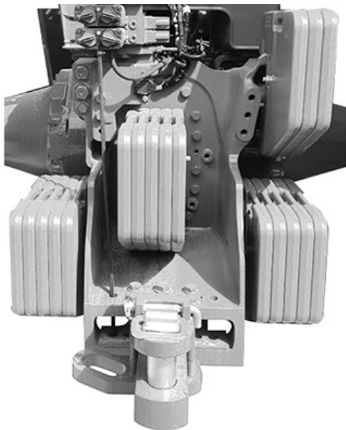
Konfigurácia maximálneho závažia bez vývodového hriadeľa a závesu
