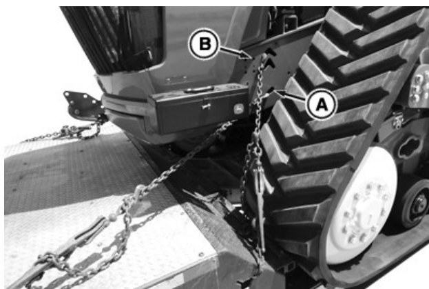
Kružok háku a drážka "T" háku (ľavá strana)
