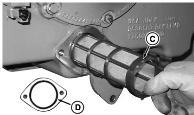
Nasávacie sito prevodovky s O-krúžkom krytu
