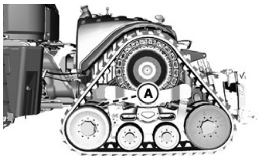
Prípojky napínacieho valca
