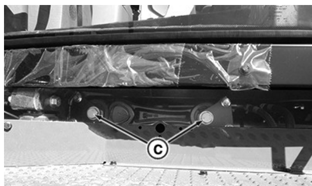
Lavá strana pod dverami kabíny
