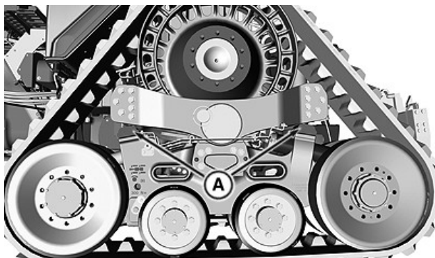
RXA0147610—UN—12MAR15 Protinárazové zarážky kĺbového spojenia podvozku
