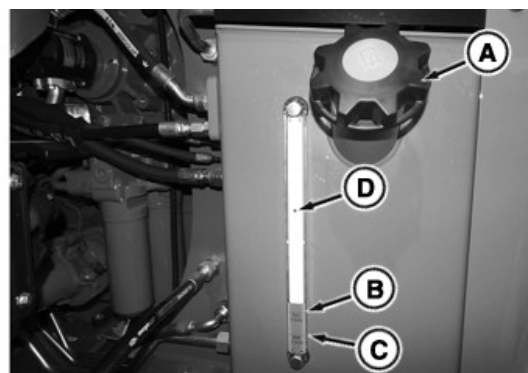
Priezor hydraulickej nádrže
