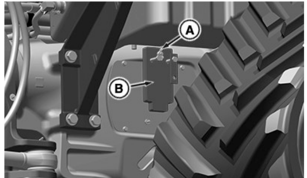
Bloccaggio dello sterzo memorizzato (lato sinistro)
