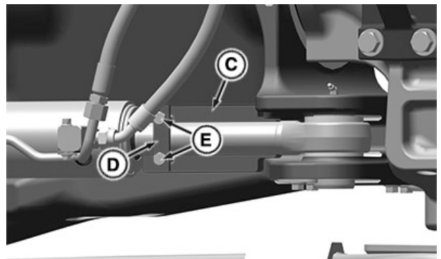
Bloccaggio dello sterzo installato (lato sinistro)
