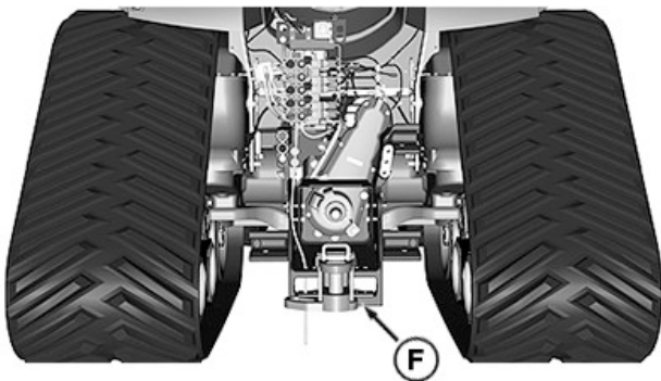
Punti di sollevamento (barra di traino posteriore)
