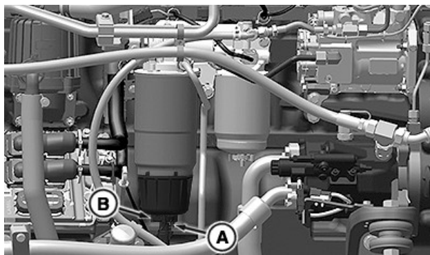
Filtro carburante, motore da 13,6 l
