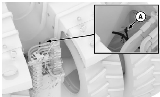
Connettore del cablaggio del sensore dello sforzo
