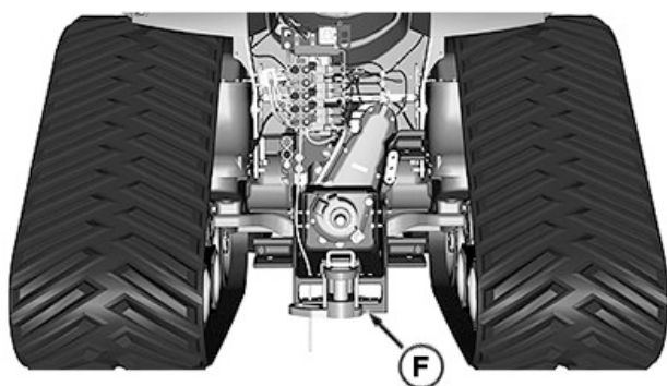
Podpěrné body (zadní spodní závěs)
