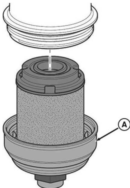
RG30727—UN—08AUG18 Montáž pouzdra řadového filtru kapaliny výfuku vznětového motoru DEF
