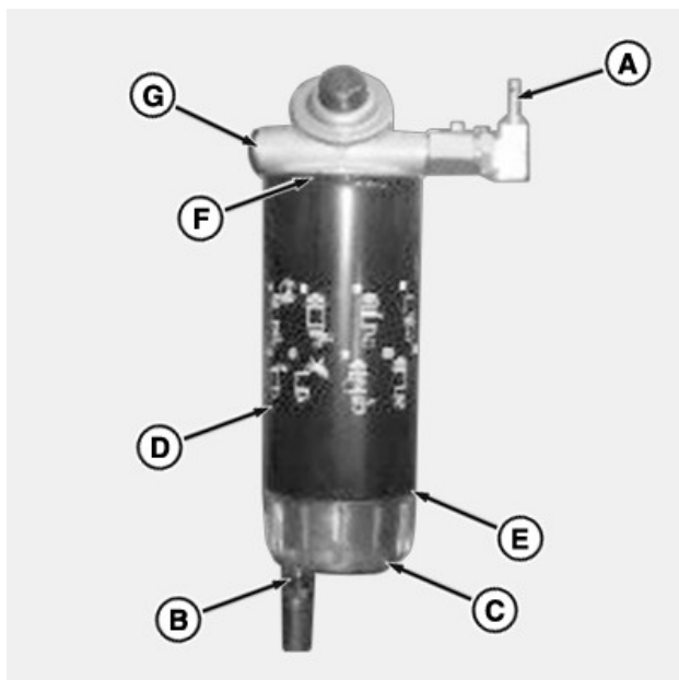
RXA0168513—UN—03JUN19 Uzávěr tlačítka plnění se může lišit
