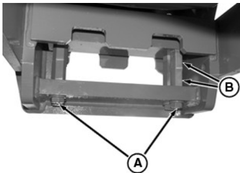
RXA0082010—UN—05JUL05 Configuration du support de barre d'attelage plus grande pour racleur
