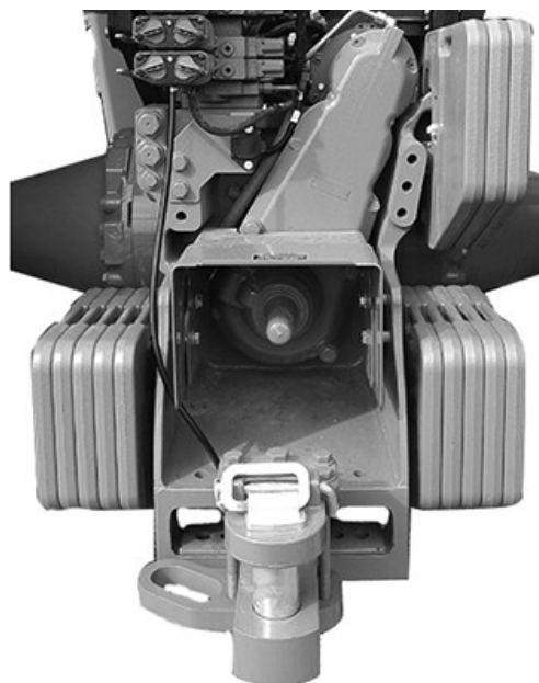
RXA0153814—UN—07SEP16 Максимална конфигурация за баласт с BOM
