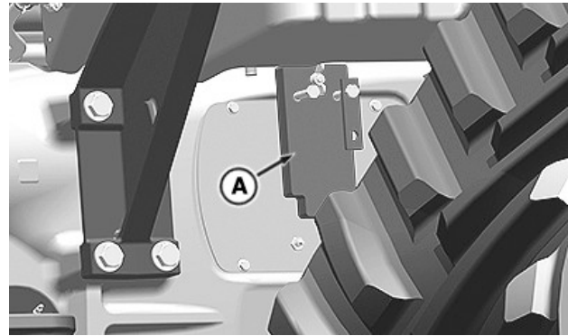
Съхранена блокировка на кормилното управление (отляво)
