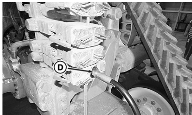
Съединение на ПУК I
