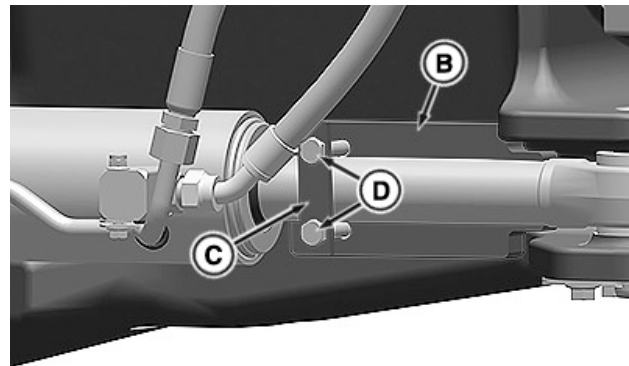
Монтирана блокировка на кормилното управление (отляво)
