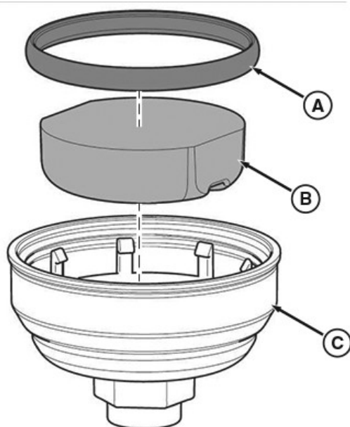
Filterhusets komponenter
