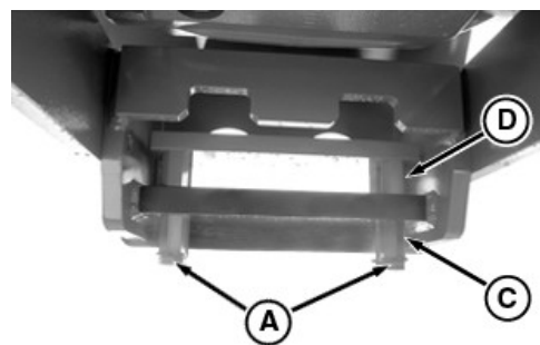
RXA0082012—UN—05JUL05 Inställning för mindre fäste till avskrapardragbom
