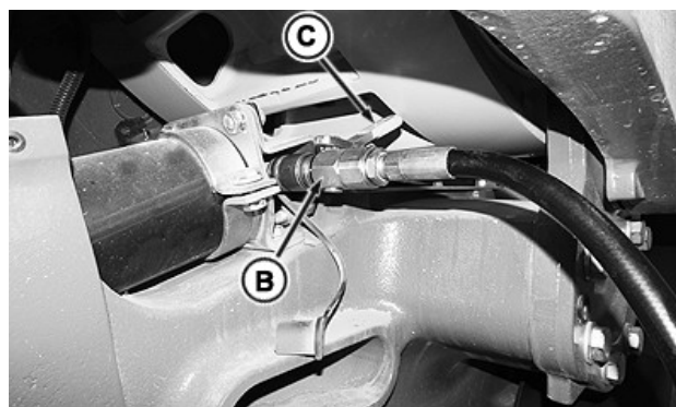
Slang, bandspänning-/slackning
