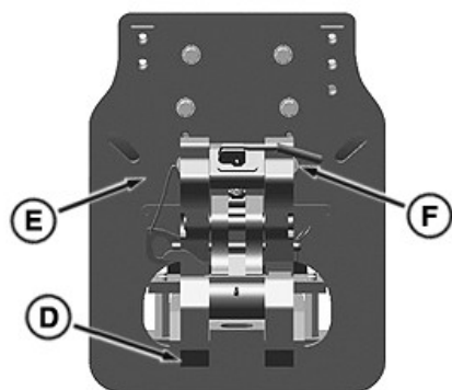
RXA0148253—UN—29MAY15 Snabbkoppling till dragbom
