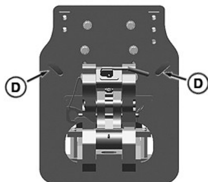
RXA0142716—UN—21JUL14 Fäste till avskrapardragbom
