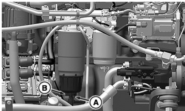
Bränslefilter för 13,6-liters motor
