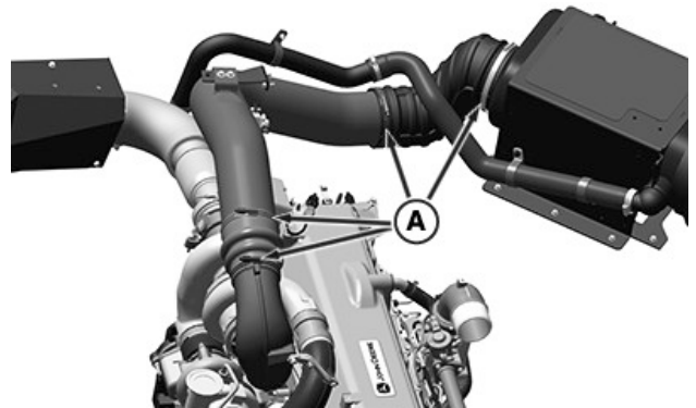
Dubbelturbomotor
