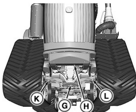
Podizne točke (prednje)
