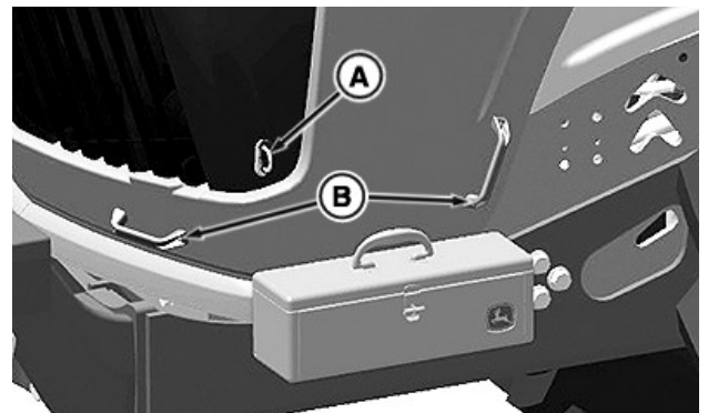
Otpuštanje poklopca motora i ručke poklopca motora
