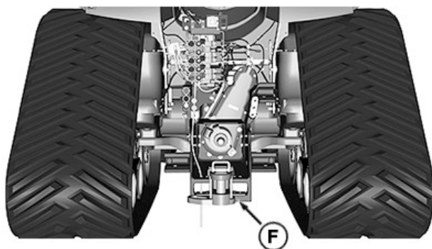
Podizne točke (stražnja ljučjajuća poteznica)
