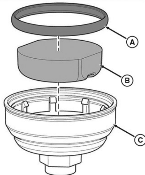
Componentele carcasei filtrului
