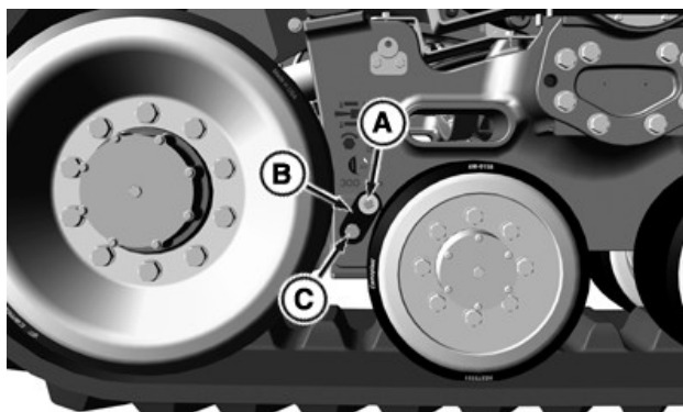
RXA0147877—UN—06APR15 Cadrul exterior al șenilei
