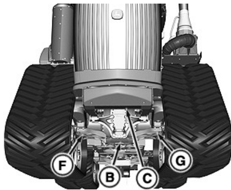
Forreste løftepunkter
