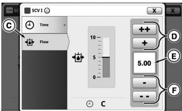
Indstilling af fjernstyreventilflow i spærrestilling
