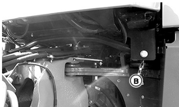
Bag ved og nede under førerhuset i højre side
