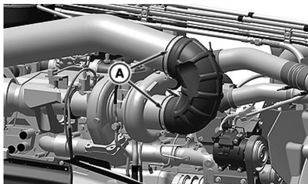
På højre side af motoren
