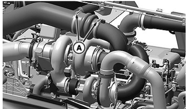
RXA0180399—UN—10NOV20 Sistema de admisión de aire—Lado derecho
