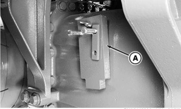
Bloqueo de bisagra almacenado en el lado izquierdo
