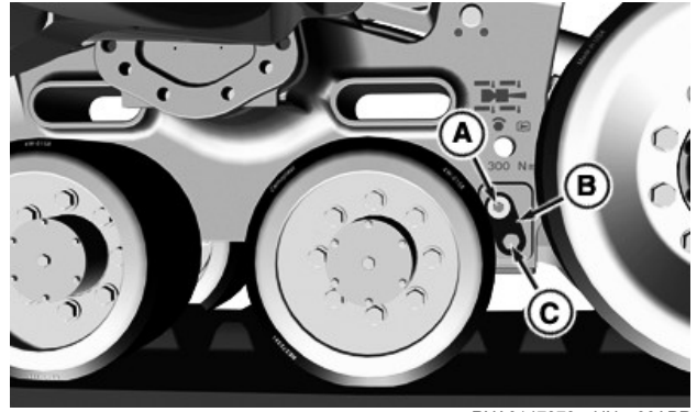
RXA0147878—UN—06APR15 Bastidor de la cadena de oruga interior
