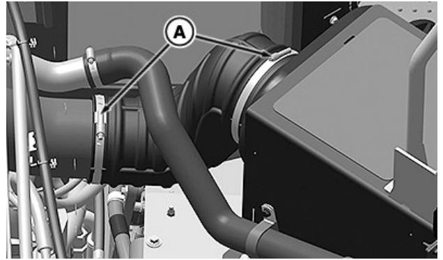
RXA0180398—UN—10NOV20 Sistema de admisión de aire—Lado izquierdo
