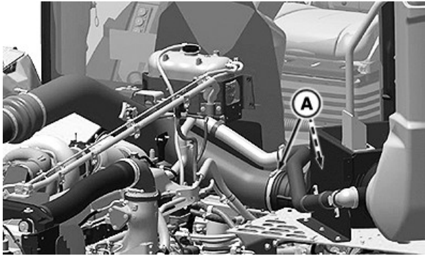
RXA0180449—UN—19NOV20 Sistema de admisión de aire—Lado izquierdo
