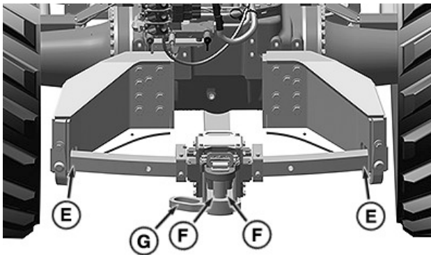
маятникового тягово-зчіпного пристрою з широким кутом повороту
