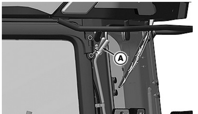
RXA0180428—UN—11NOV20 Фільтр системи вентиляції бака для сечовини (A) знаходиться вгорі лівого заднього кута кабіни.
