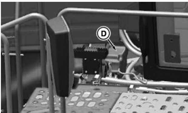
Панель головних плавких запобіжників (D) знаходиться з лівого боку задньої сторони нижньої опори капоту.
