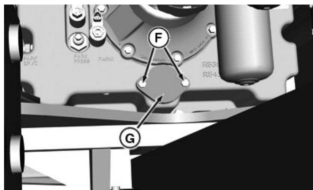
Вигляд трансмісії PowerShift ззаду
