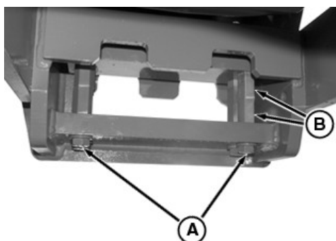
RXA0082010—UN—05JUL05 Configuration du support de barre d'attelage plus grande pour racleur
