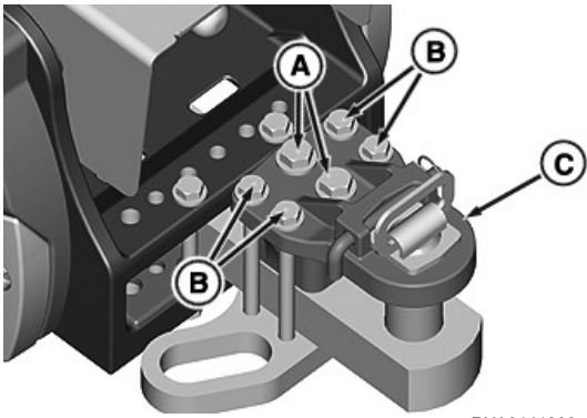
RXA0141899—UN—05JUN14 Barre d'attelage renforcée
