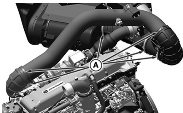
Motor cu turbosufiantă cu o singură treaptă
