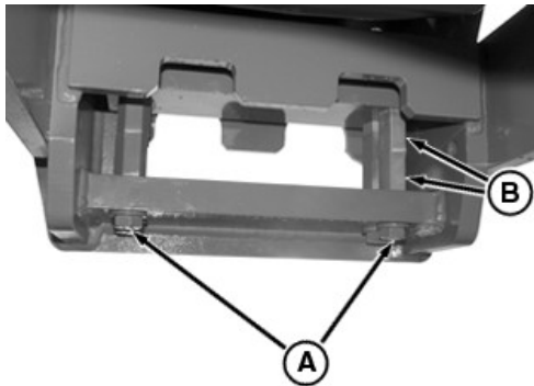
RXA0082010—UN—05JUL05 Configurarea suportului barei de tractare mai mari a screperului
