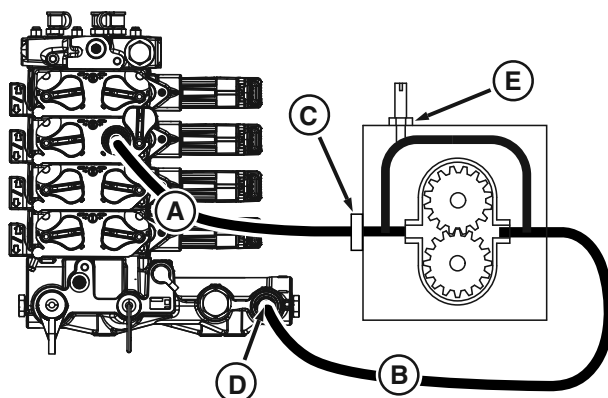
Pompă de stopire—fără cuplaj
