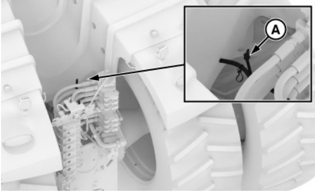
RX1405634—UN—23MAY25 Conectarea cablajului senzorului de tracțiune
