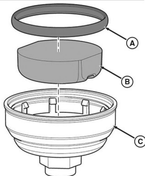
Szűrőház alkatrészei
