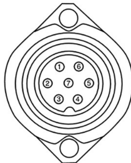
ISO 11786 kimenet rajz
