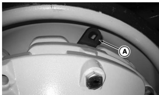
JDG10958 Keréksúly tartó kulcs
