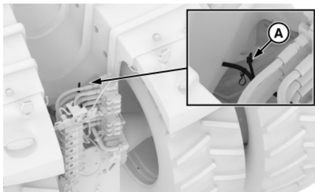
Erzékelő kábelköteg csatlakozója
