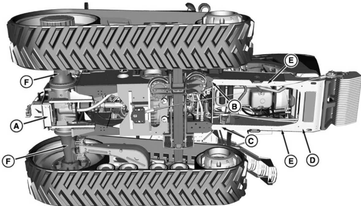
Punti di sollevamento parte inferiore
