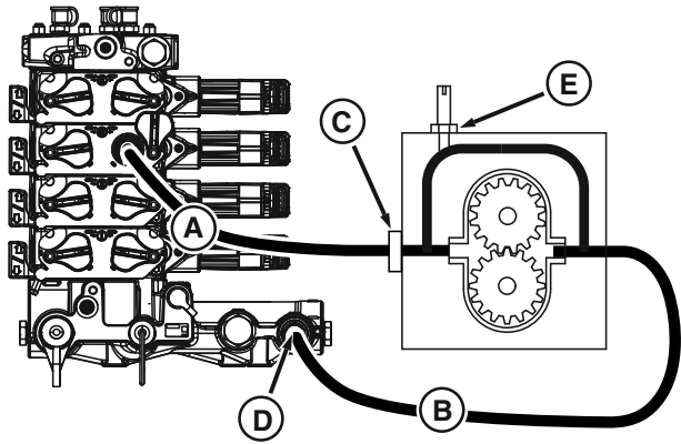
Pompa per l'irrigazione—Senza sollevatore RXA0188469—UN—25JAN23
