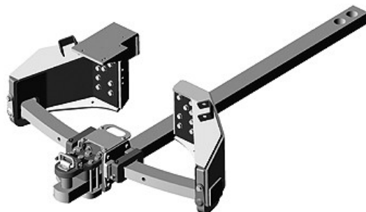
Supporto barra di traino ad ampia oscillazione, portata 4580 kg (10100 lb)
