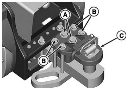
Barra di traino per impiego gravoso
