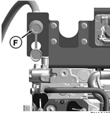
F—Attacco della coppa (scarico della scatola motore)
