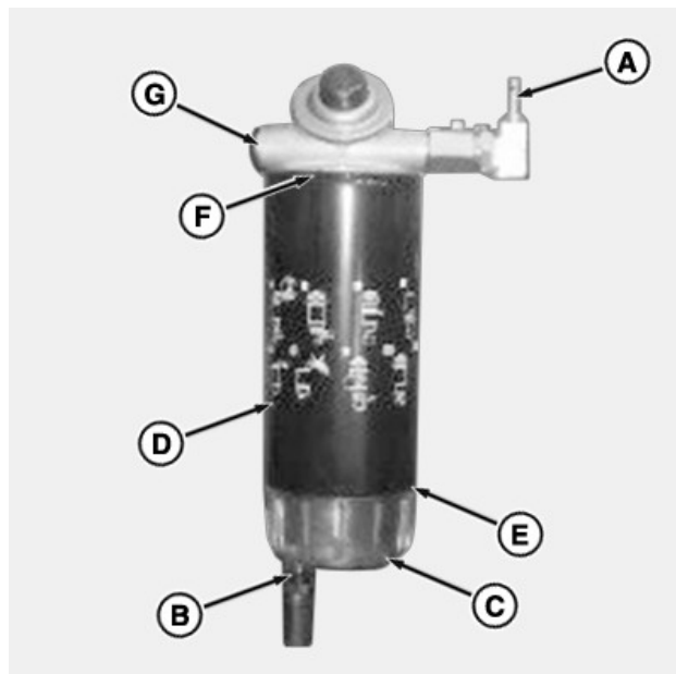
RXA0168513—UN—03JUN19 Il cappuccio del pulsante di adescamento può essere diverso
