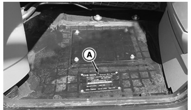
La targhetta del numero di serie della cabina (A) si trova sotto il tappetino del pavimento della cabina in corrispondenza della portiera
