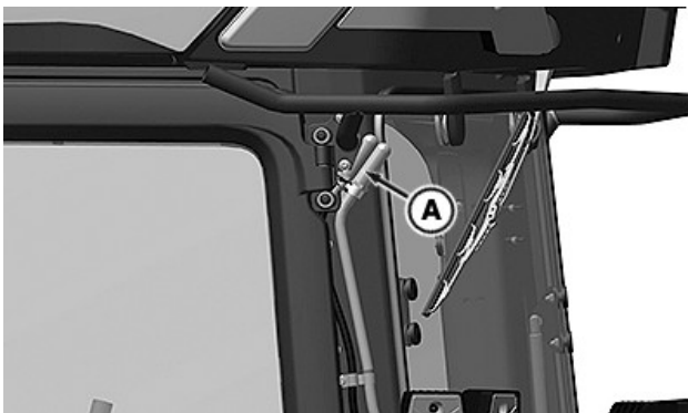
RXA0180428—UN—11NOV20 Il filtro di sfiato del serbatoio DEF (A) è vicino alla parte superiore dell'angolo posteriore sinistro della cabina.
