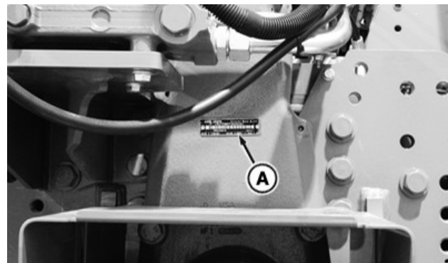
Il numero di serie della scatola di riduzione della PTO (A) si trova sulla scatola di riduzione della PTO sul lato posteriore del trattore
