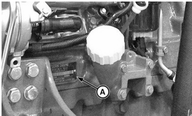
Targhetta del numero di serie del motore (A) (componenti rimossi per chiarezza)
