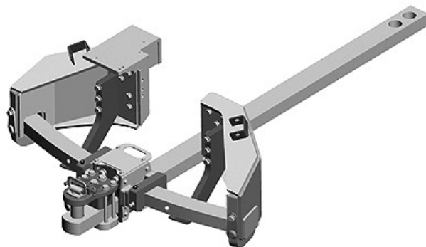
Supporto barra di traino ad ampia oscillazione con kit di supporto ad alta portata, portata 5440 kg (12000 lb)
