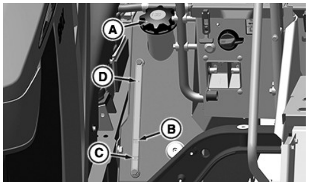
Spia trasparente olio idraulico/trasmissione
