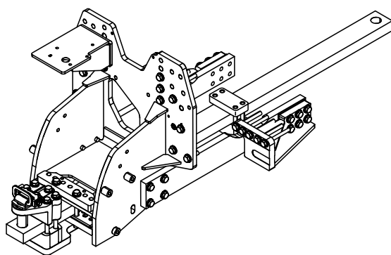
Supporto barra di traino rinforzata, capacità 4990 kg (11000 lb)
