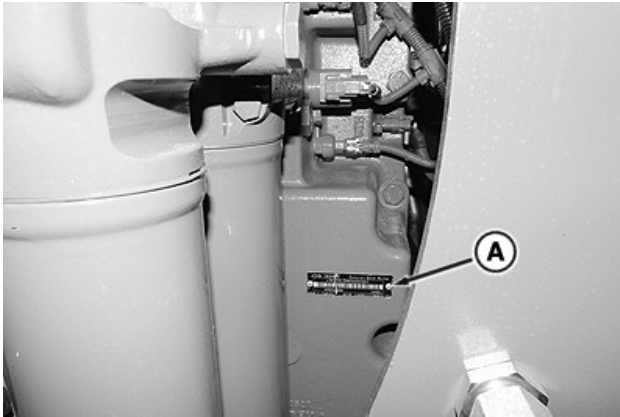
Il numero di serie della trasmissione (A) si trova sul lato posteriore destro della scatola della trasmissione (vicino ai filtri della trasmissione)
