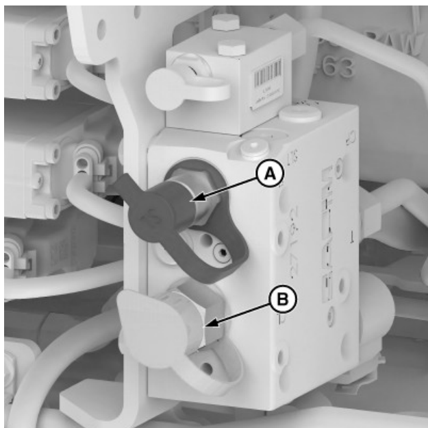
Attacco freno idraulico del rimorchio
