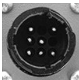
Connettore ISO 11783
